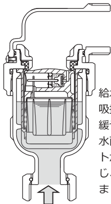
充水時（弁閉止時）
