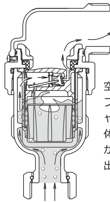
自動空気抜き時（排気時）
